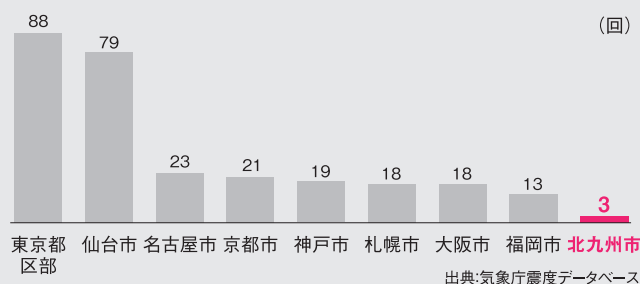
震度4以上の地震の回数(過去100年)
